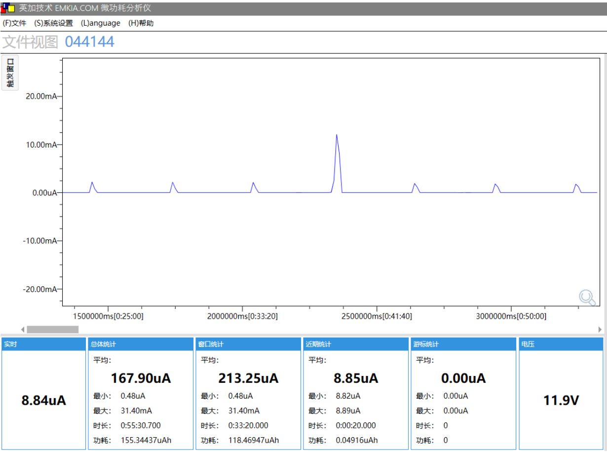
图 1 功耗分析图
