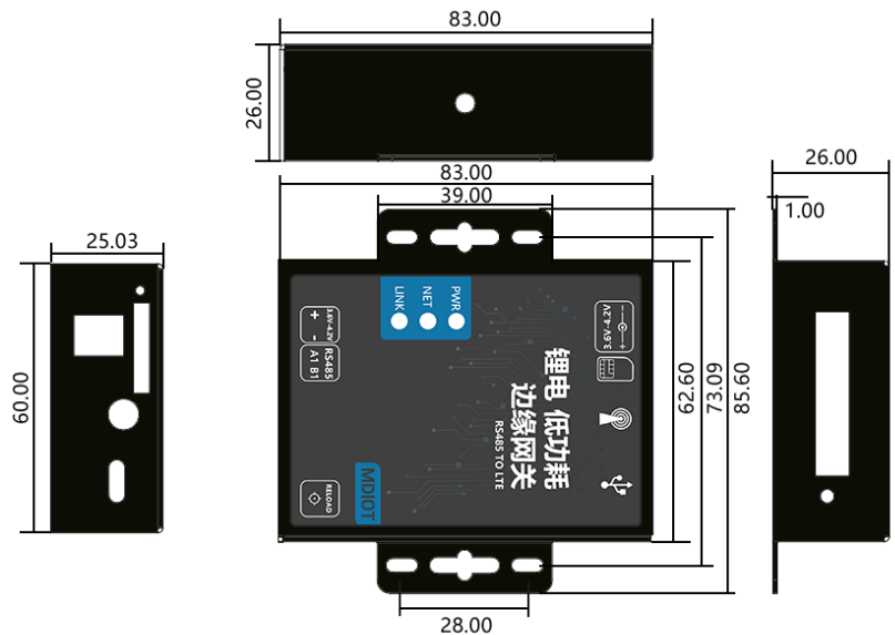
图 3 低功耗 DTU 机械尺寸图 (TOP View)
