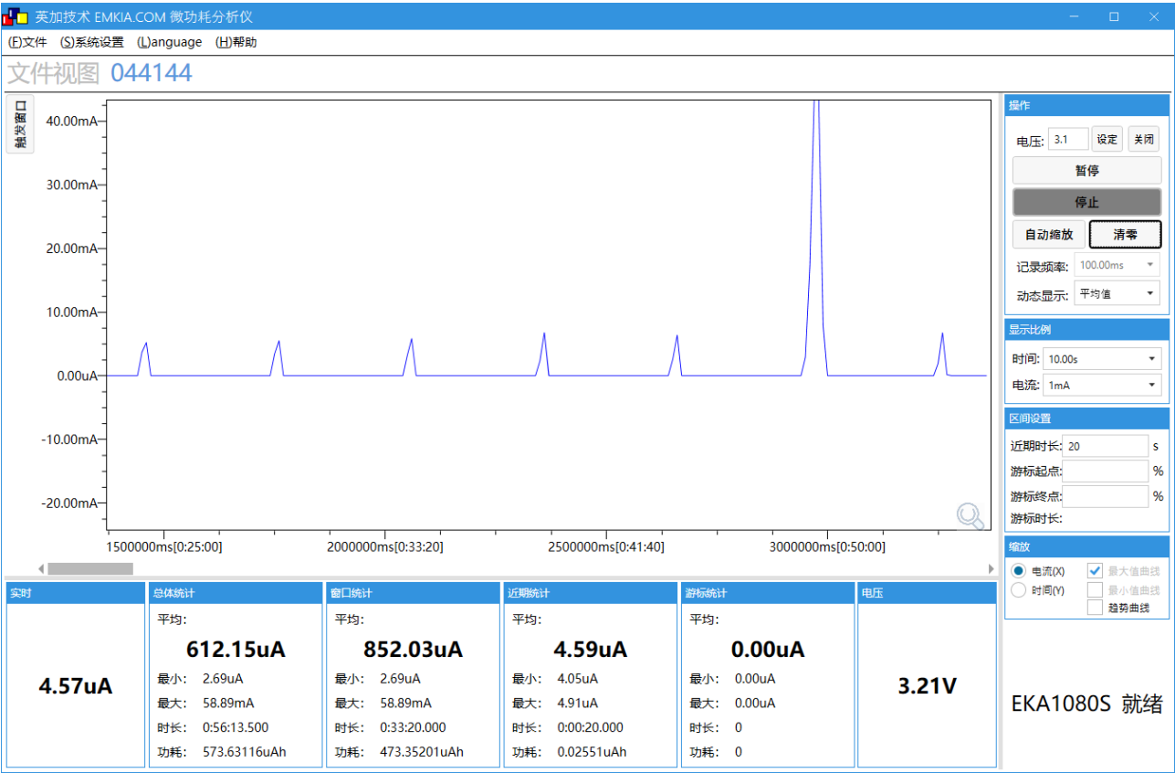
图 1 功耗分析图
