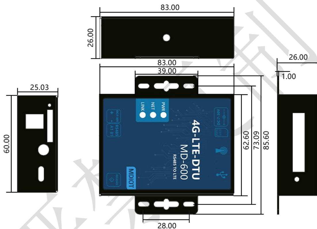
图 2 MD600 DTU 尺寸图
