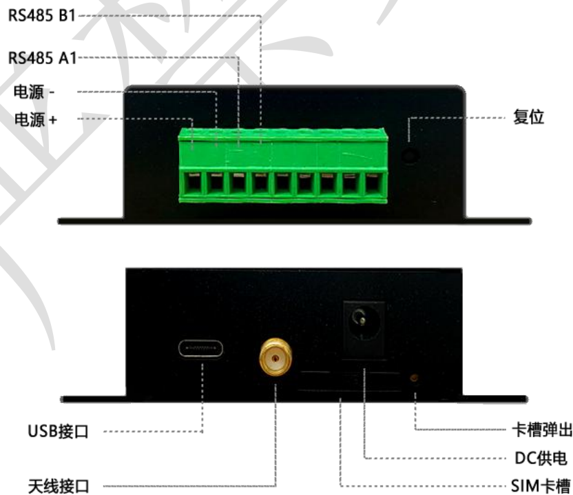
图 1 MD600 DTU 插针引脚图
