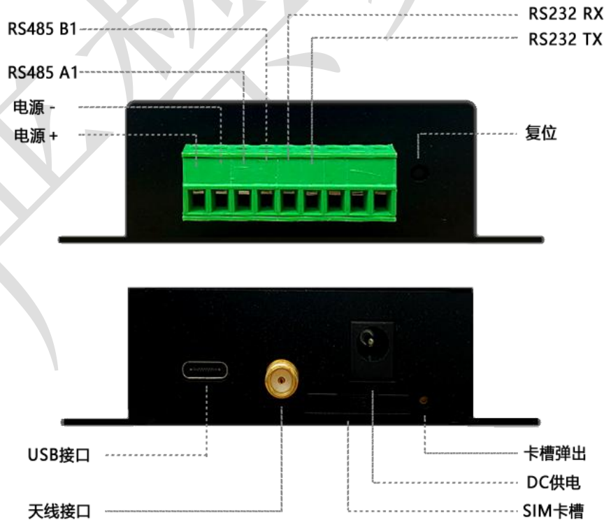
图 1 MD606 DTU 插针引脚图
