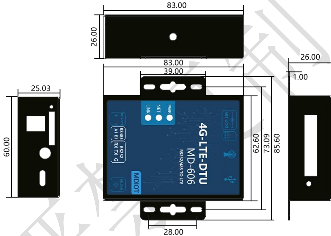
图 2 MD606 尺寸图
