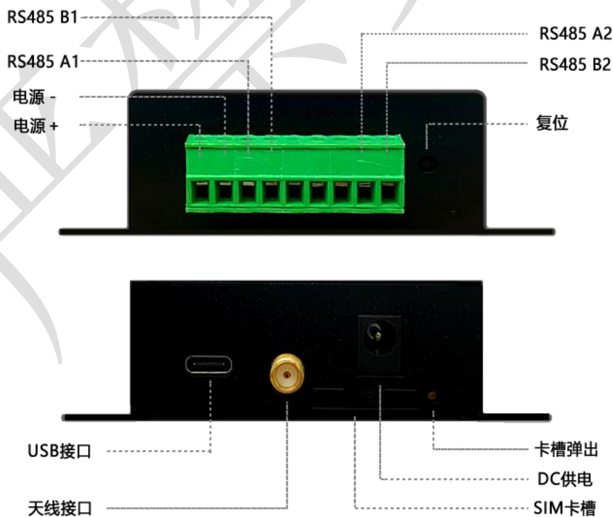
图 1 MD608 DTU 插针引脚图
