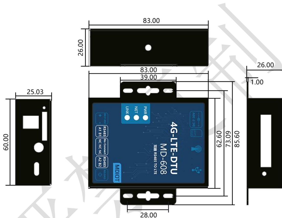
图 2 MD60 尺寸图
