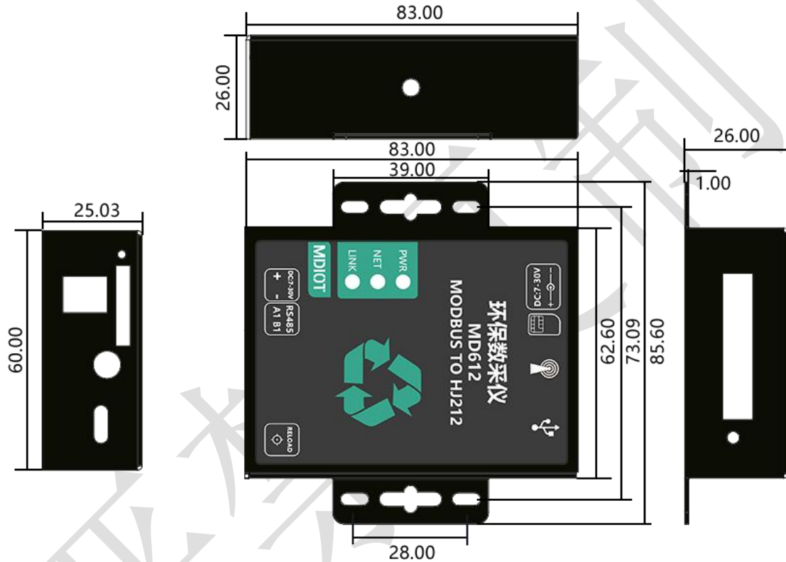
图 2 MD612 环保网关尺寸图
