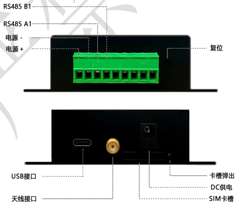
图 1 MD612 环保网关插针引脚图
