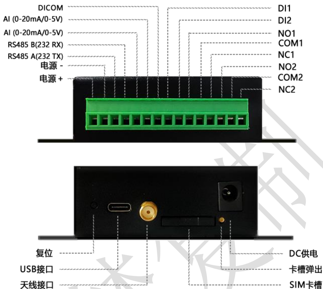
图 1 MD620 RTU 插针引脚图
