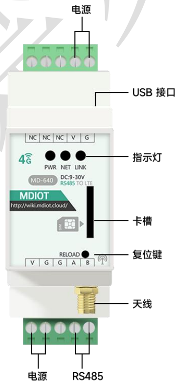
图 1 MD640 DTU 插针引脚图
