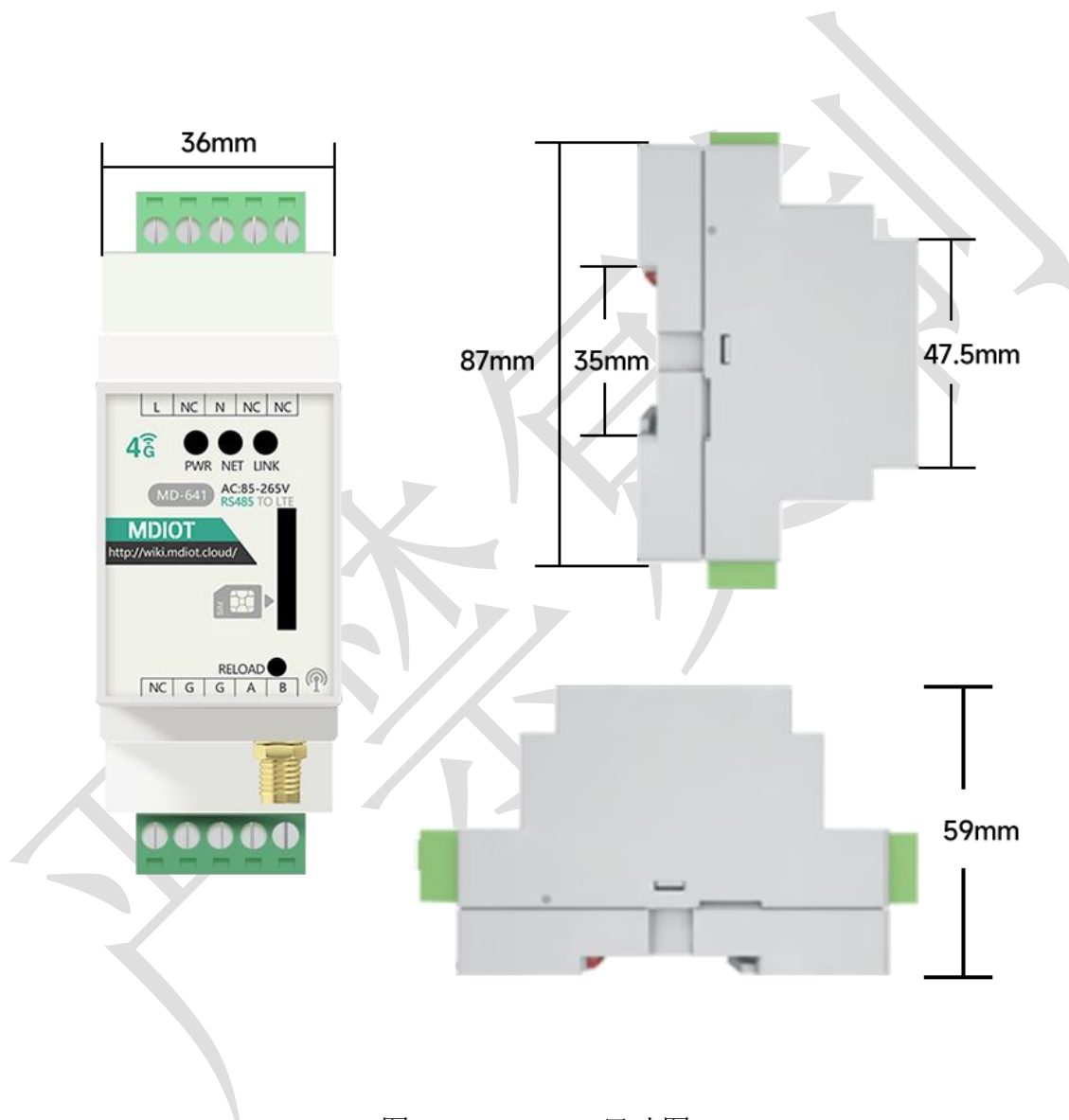
图 2 MD641 DTU 尺寸图
