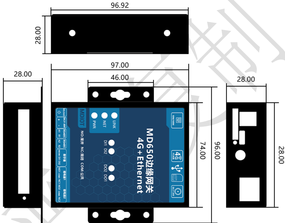
图 2 MD650 DTU 尺寸图
