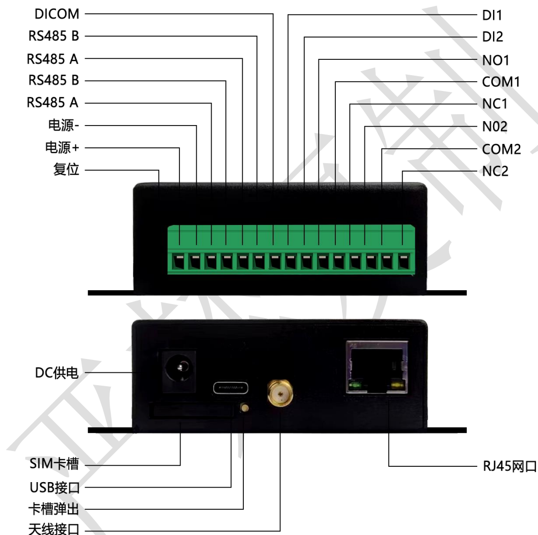
图 1 MD655 RTU 插针引脚图
