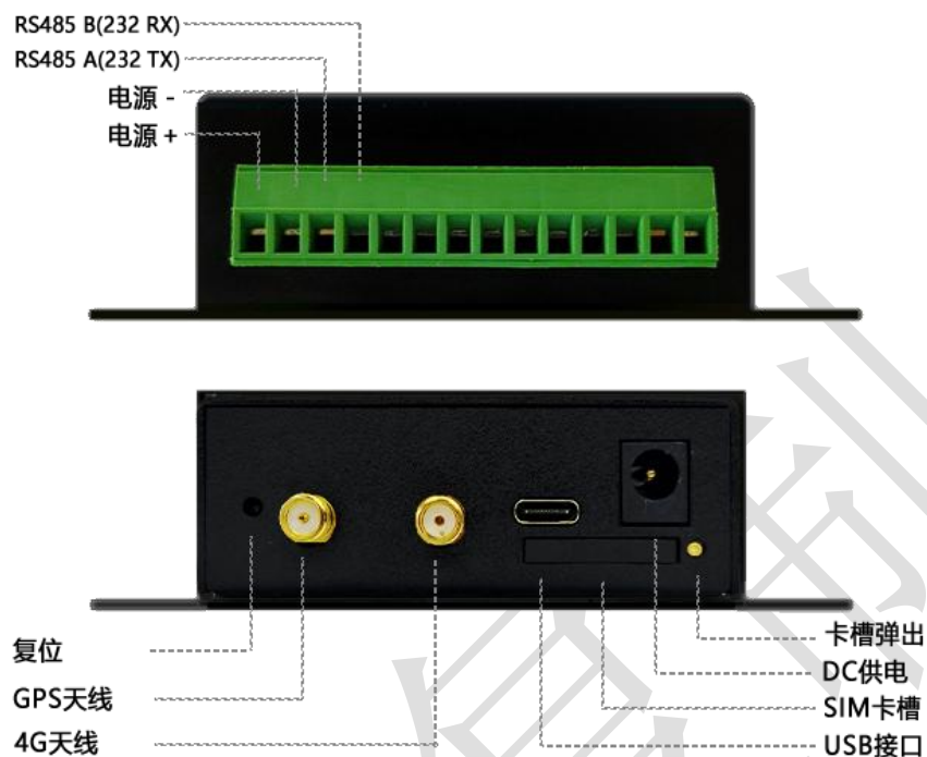
图 1 MD662 DTU 插针引脚图
