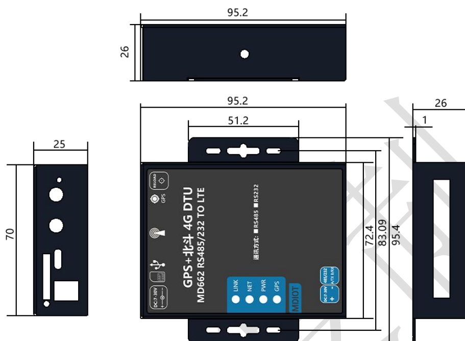
图 2 MD662 DTU 尺寸图
