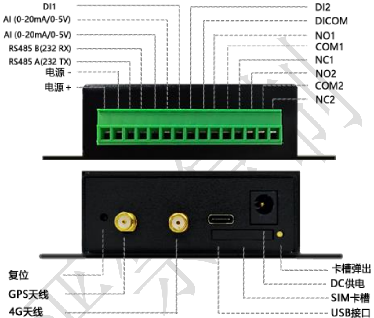
图 1 MD663 RTU 插针引脚图
