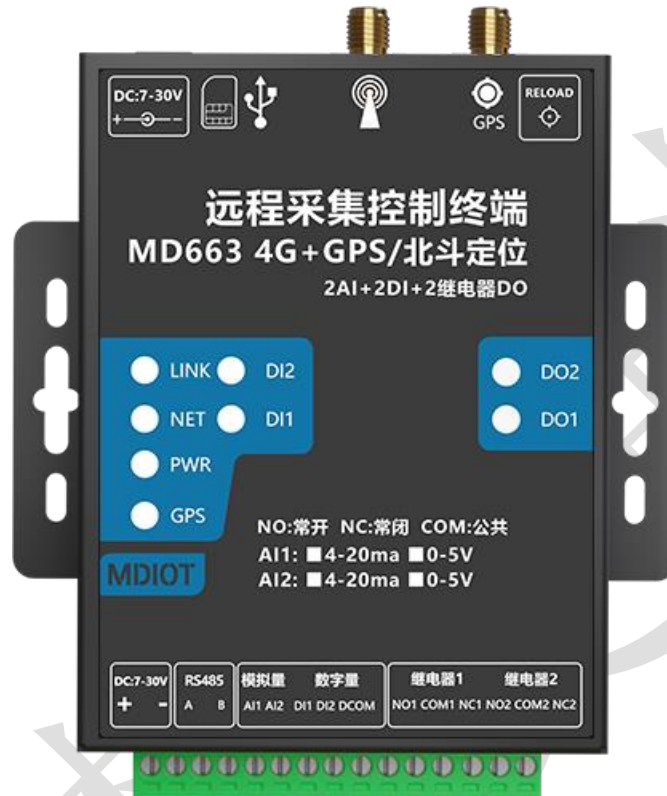
图 3 MD663 RTU 实物图
