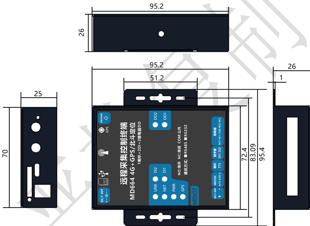
图 2 MD664 RTU 尺寸图
