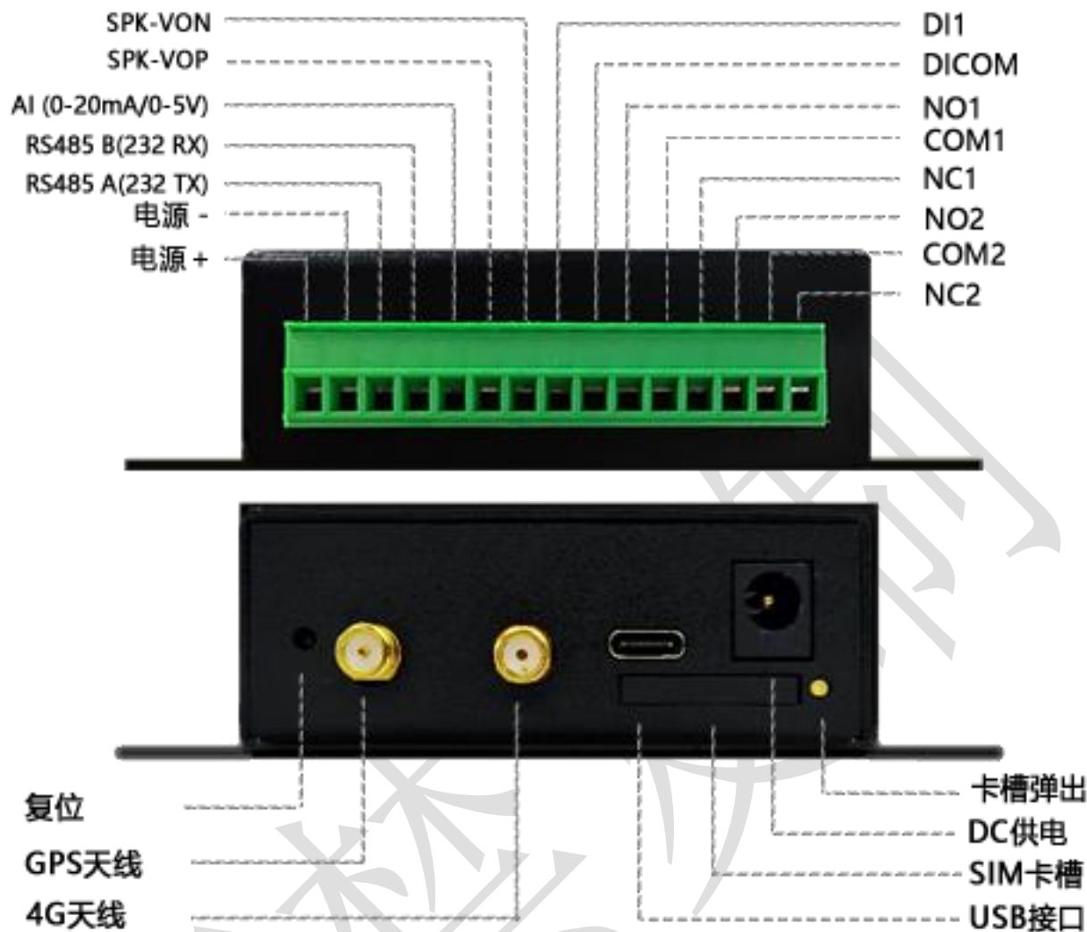
图 1 MD664 RTU 插针引脚图
