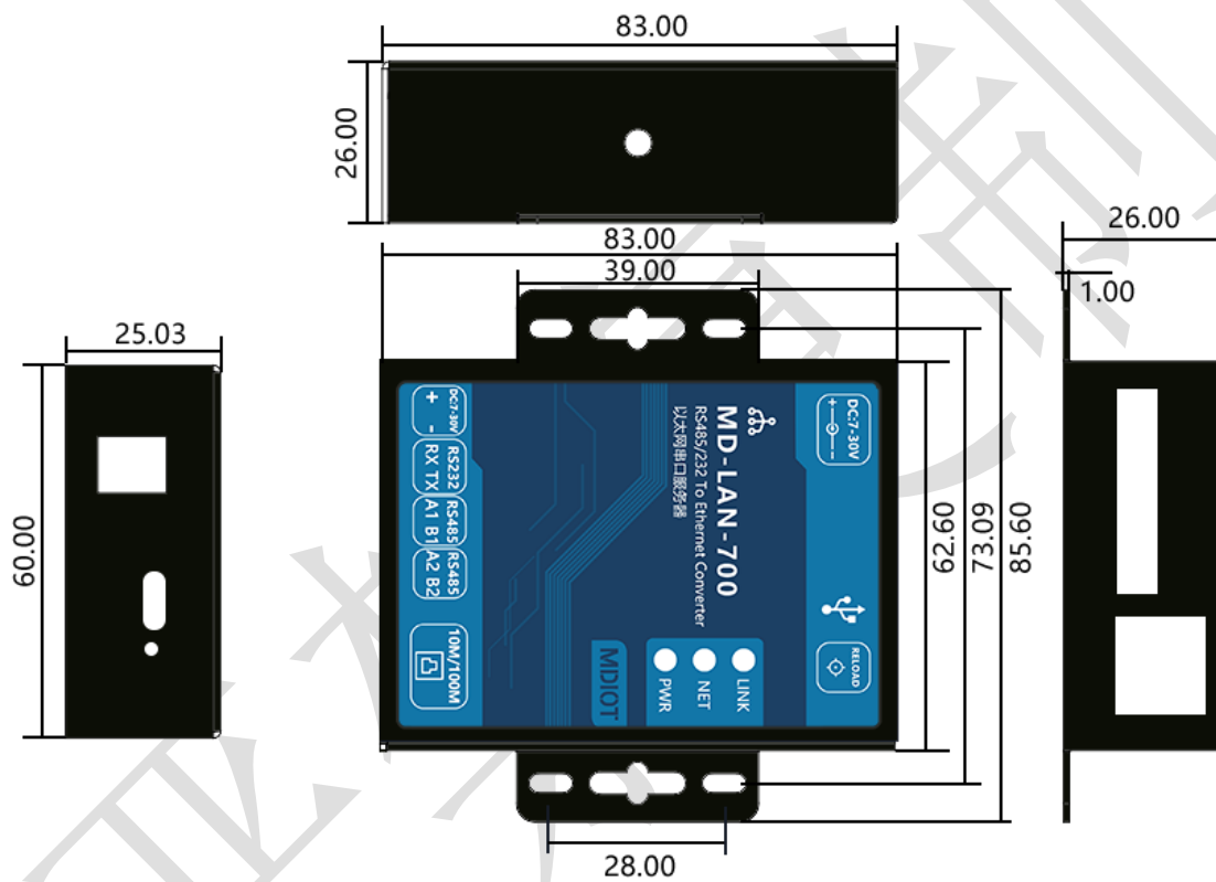
图 2 MD700 DTU 尺寸图
